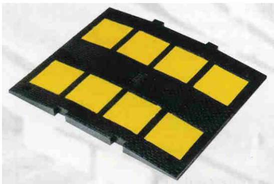
Modulo F.to cm.48x60x3 Terminale Maschio/Femmina F.to cm.23,5 x 60 Tassello di fissaggio mm.10 x 100
